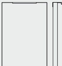
drzwi z uchwytem zintegrowanym, z obrzeżem
