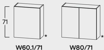
szafki wiszące, głębokość 32 cm
