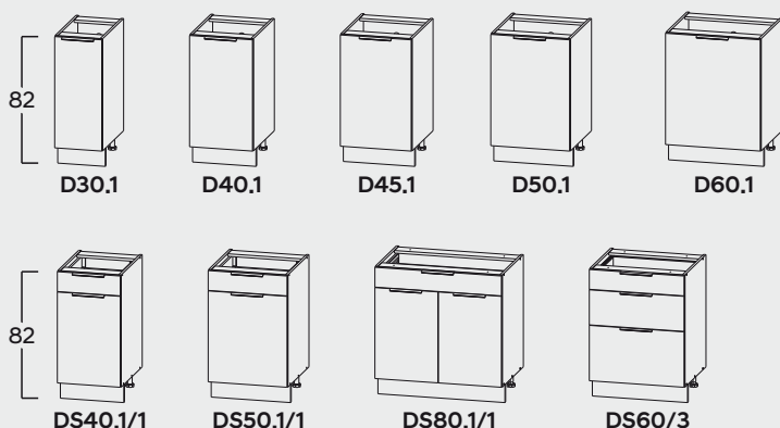
szafki dolne, głębokość 51 cm
