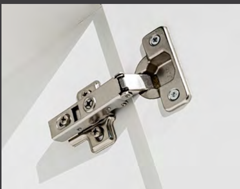
Zawiasy z cichym domykiem, regulowane w trzech płaszczyznach.
